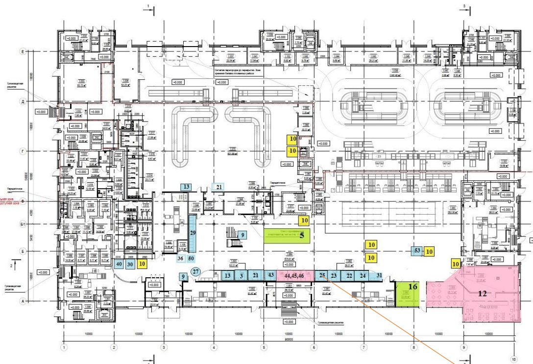
План 1-го этажа (на отм. 0.000), М 1:200
